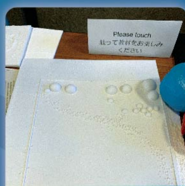
凸字赫羅圖
