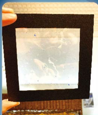
尋找小行星
